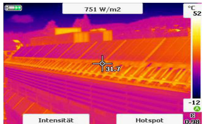
La radiación solar en W/m 2 se memoriza en cada termografía.
