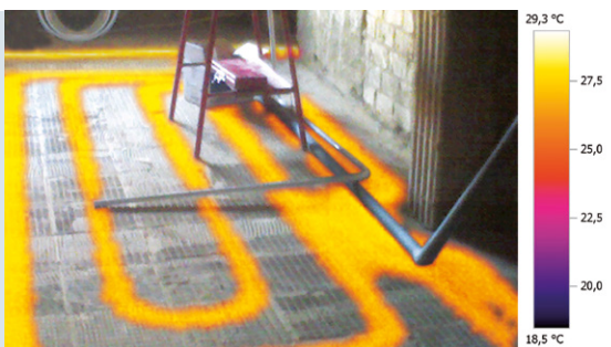
Verborgen leidingen met TwinPix ook in het echte beeld herkennen
