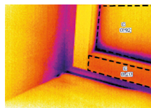
Emissiegraadverandering per bereik voor een exacte temperatuuranalyse
