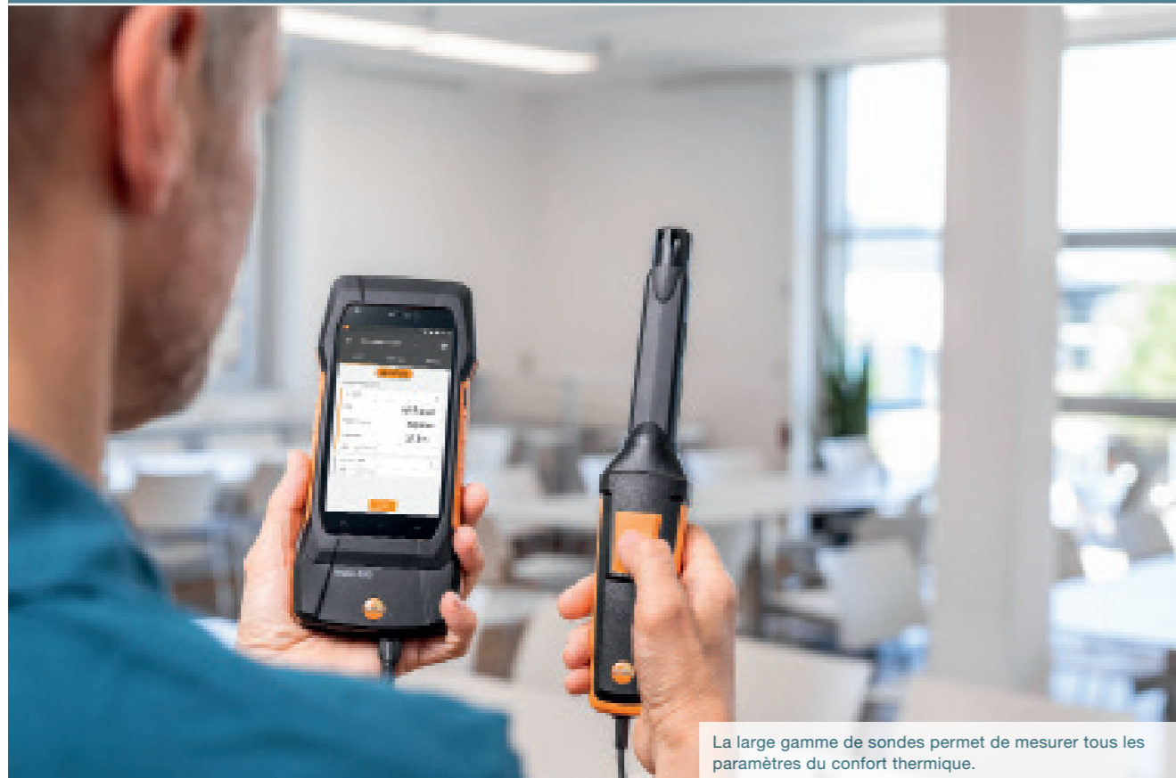
Sonde de mesure du degré de turbulence
