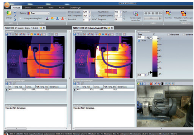
Auswertung und Vergleich mehrerer Wärmebilder sowie dem dazugehörigem Echtbild in der Software testo IIRSoft.
