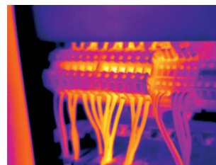
Fehlerhafte elektrische Bauteile erkennen.
