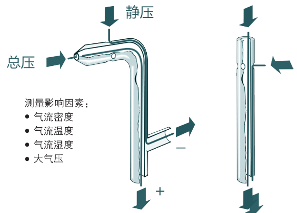
皮托管
