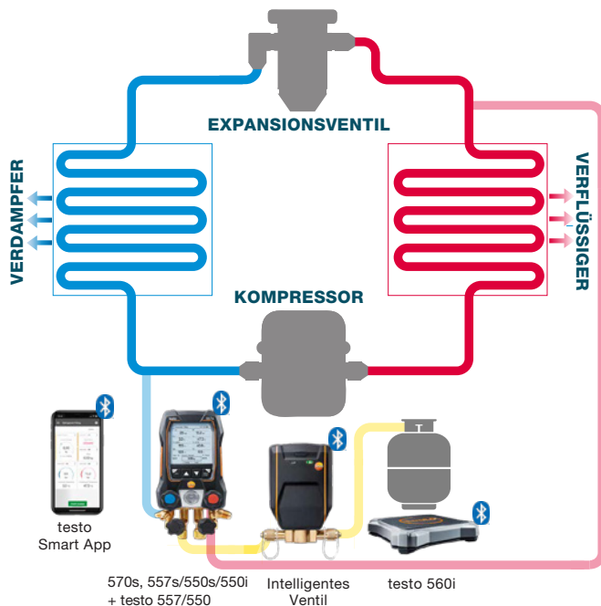
Schema für automatische Kältemittelbefüllung
